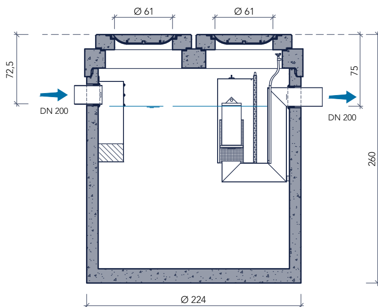
doorsnede
